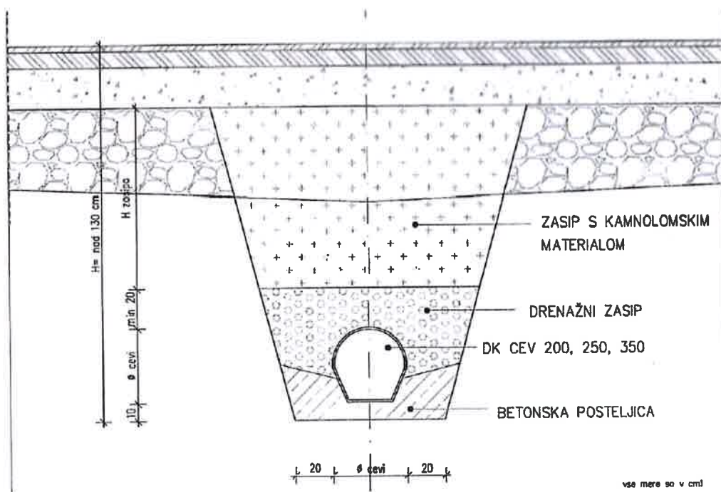
detajl izvedbe drenaže
