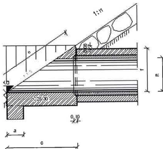
Vzdolžni prerez vtočne oz. iztočne glave
